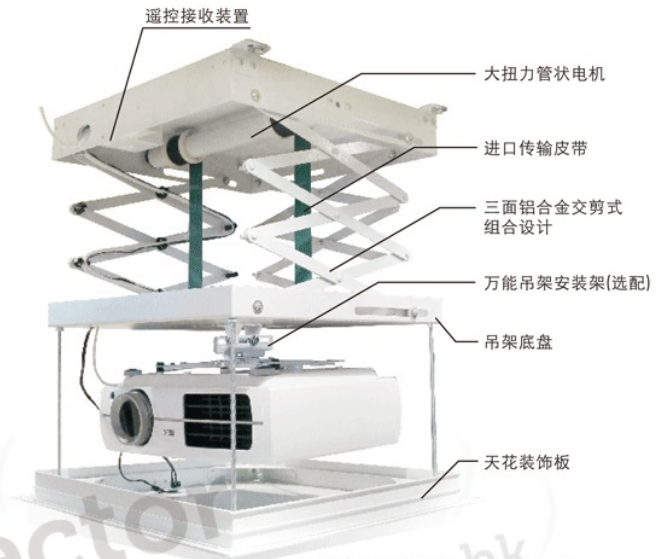
展開示意图(投影机不属于产品内)
