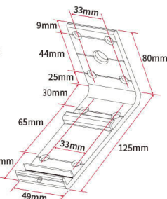
機箱掛勾
