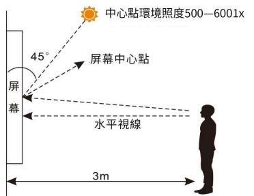
圖1 側視圖
