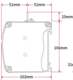
機箱側視圖
