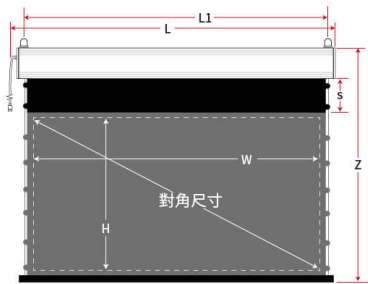
屏幕主視圖(實際投影面積在虛線內)
