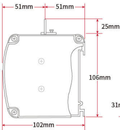
機箱側視圖
