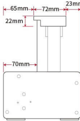
機箱側視圖(頂蓋尺寸)
