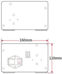
機箱側視圖
