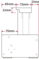
機箱側視圖(頂蓋尺寸)
